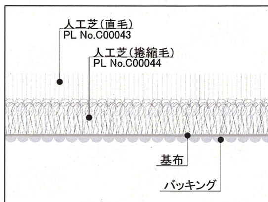
断面図（標準タイプ）
